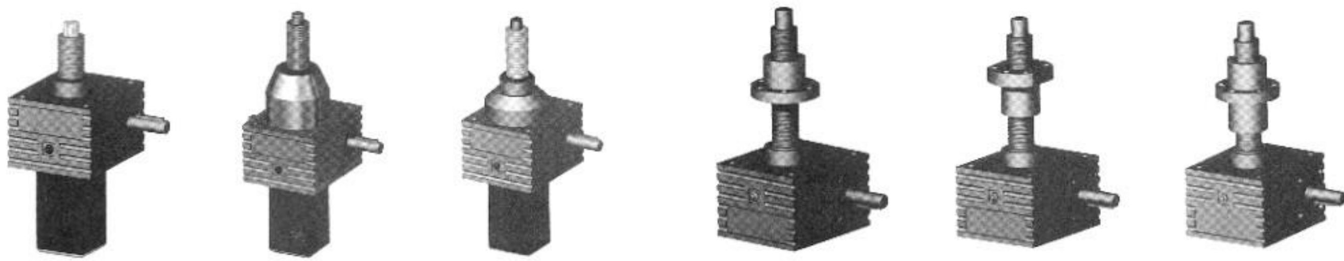
普通齿 滚珠丝杠 反齿隙 普通齿 滚珠丝杠 反齿隙
